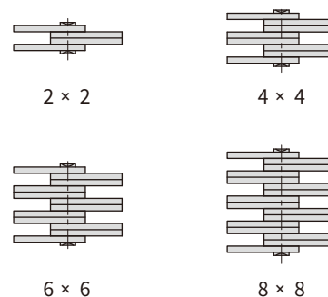
链板组合 Plate lacing
