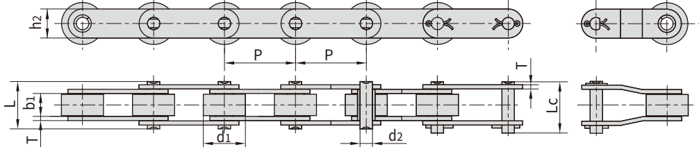
大滚子型 Large Roller Type
